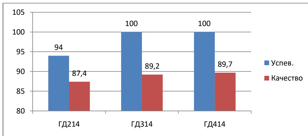
Анализ качества обучения по курсам 43.02.10 Туризм
